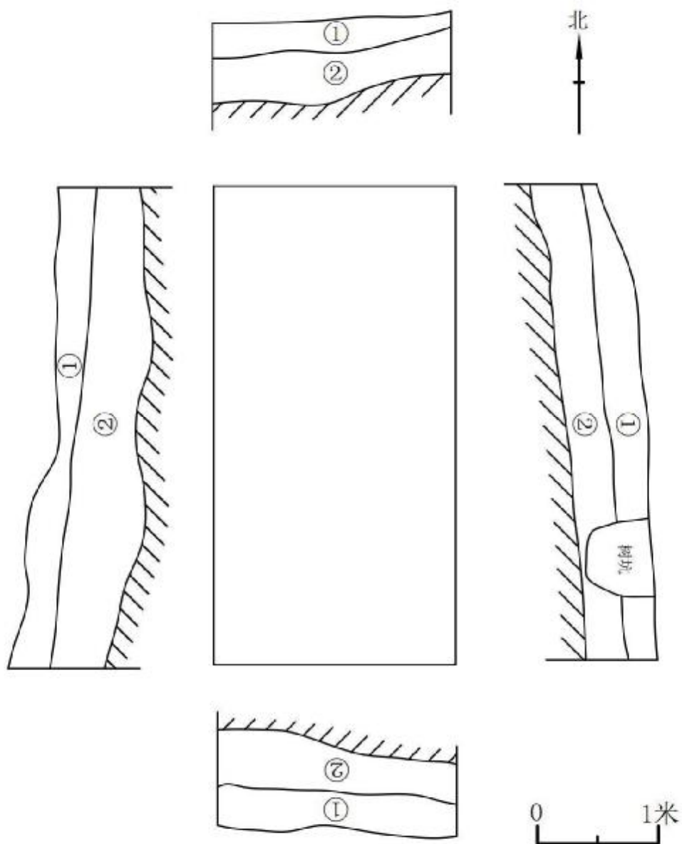
图 126 TG2 平剖面图
