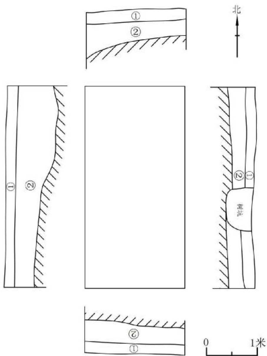
图 134 TG3 平剖面图
