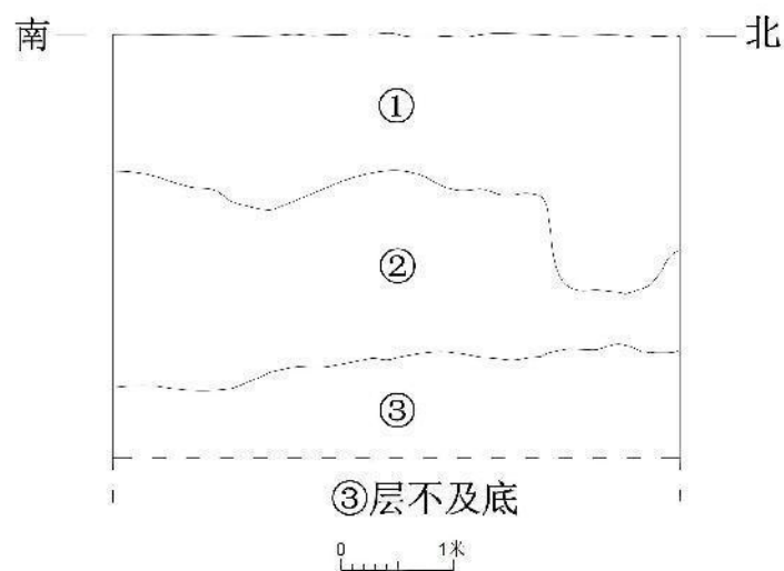
图 70 DM4 剖面图
