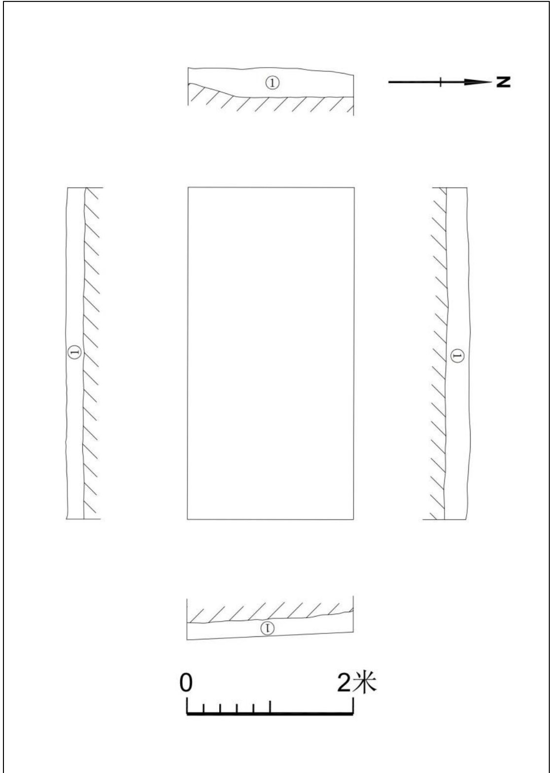
图 61 TG1 平剖面图
