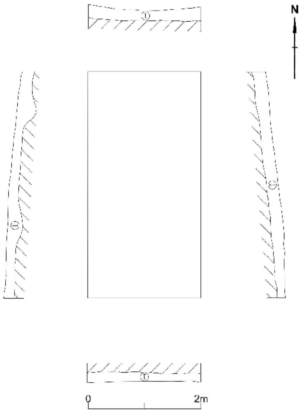
图 150 TG3 平剖面图
