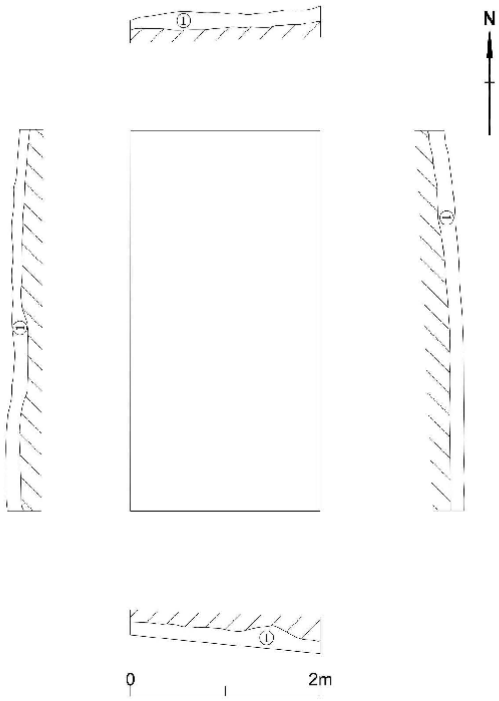
图 142 TG2 平剖面图
