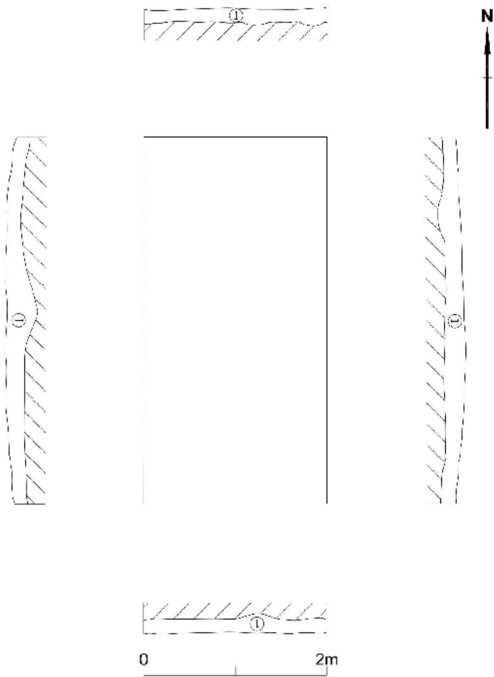
图 182 TG7 平剖面图
