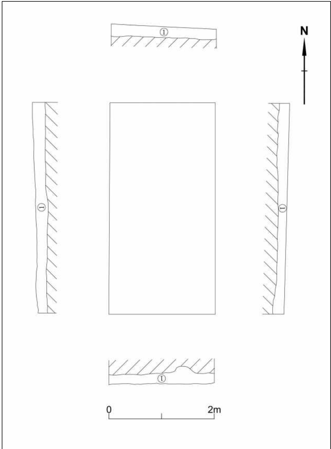
图 66 TG1 平剖面图
