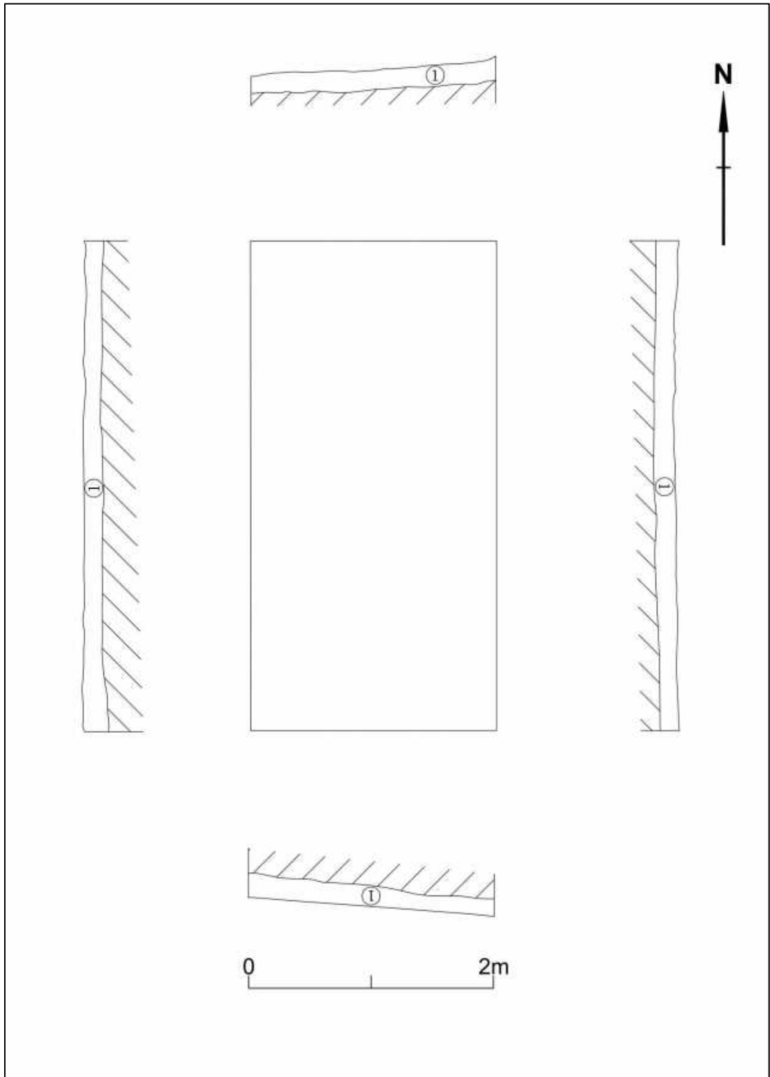
图 74 TG2 平剖面图
