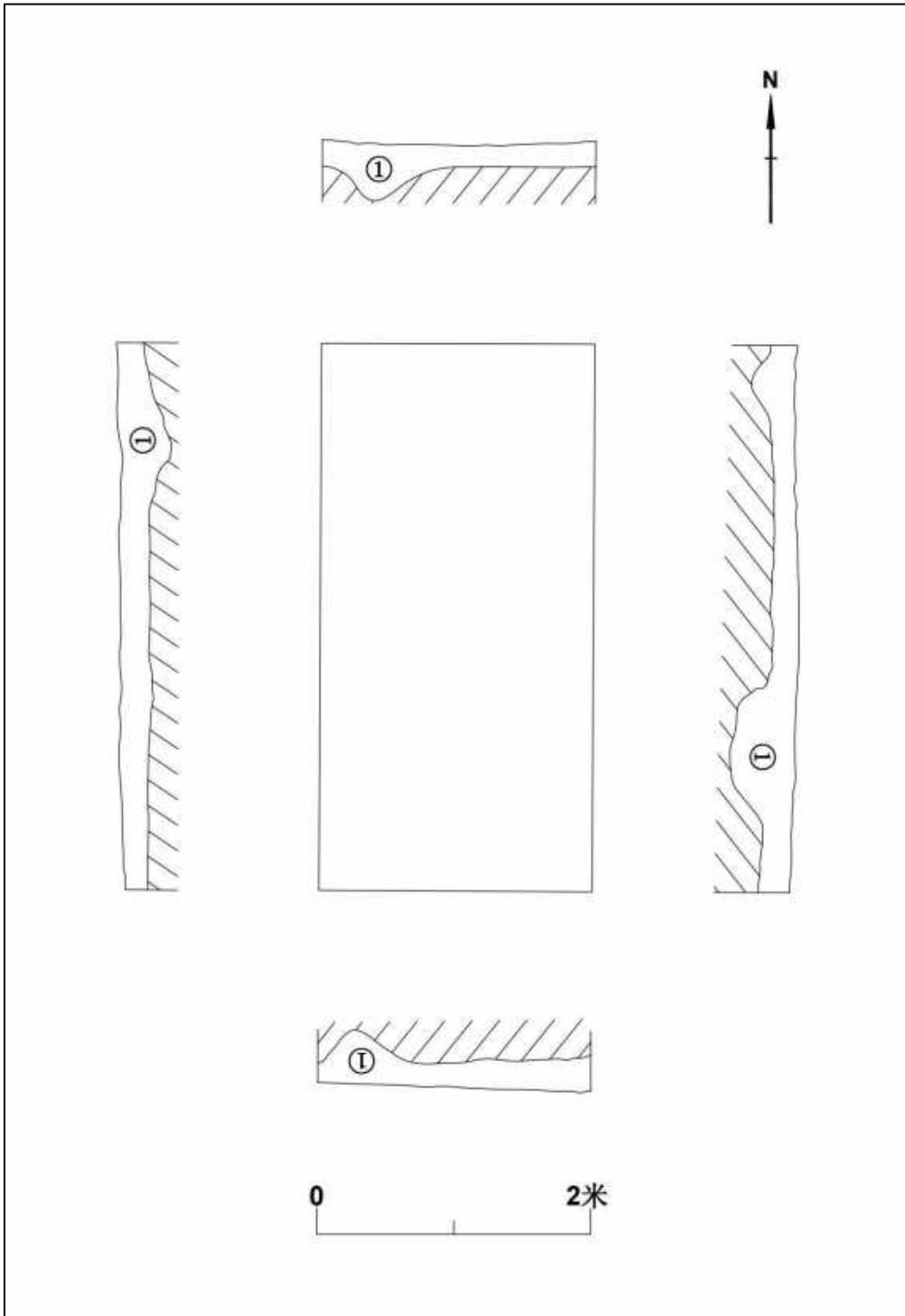
图 70 TG1 平剖面图
