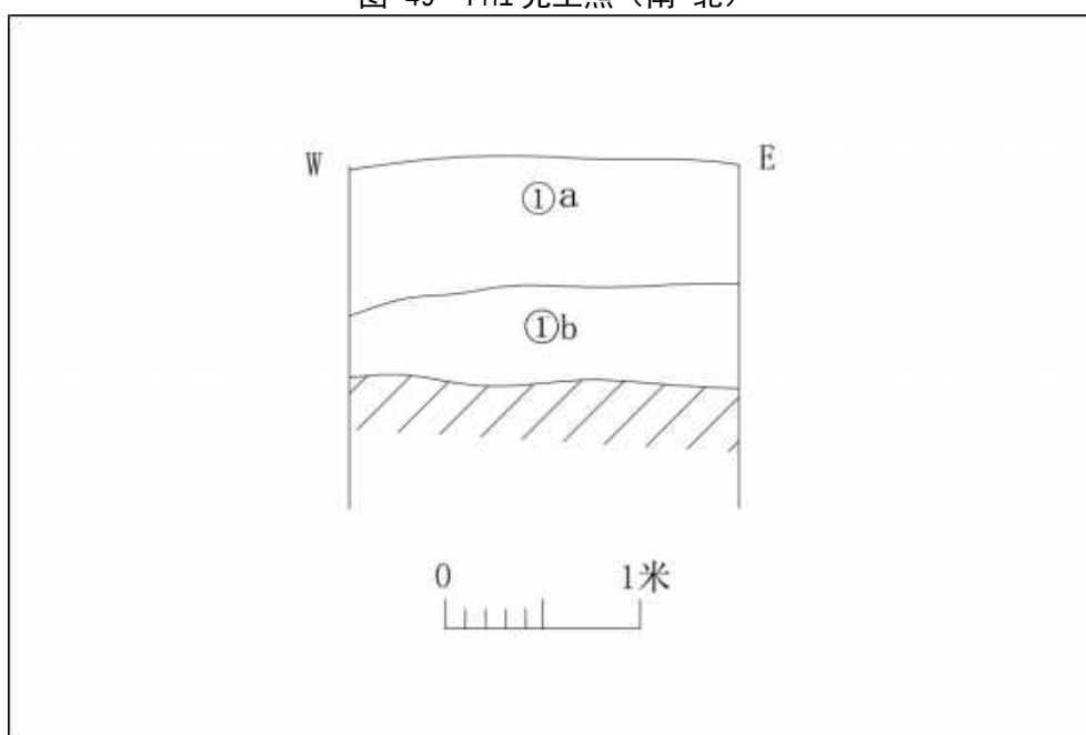
图 50 PM1 剖面图
