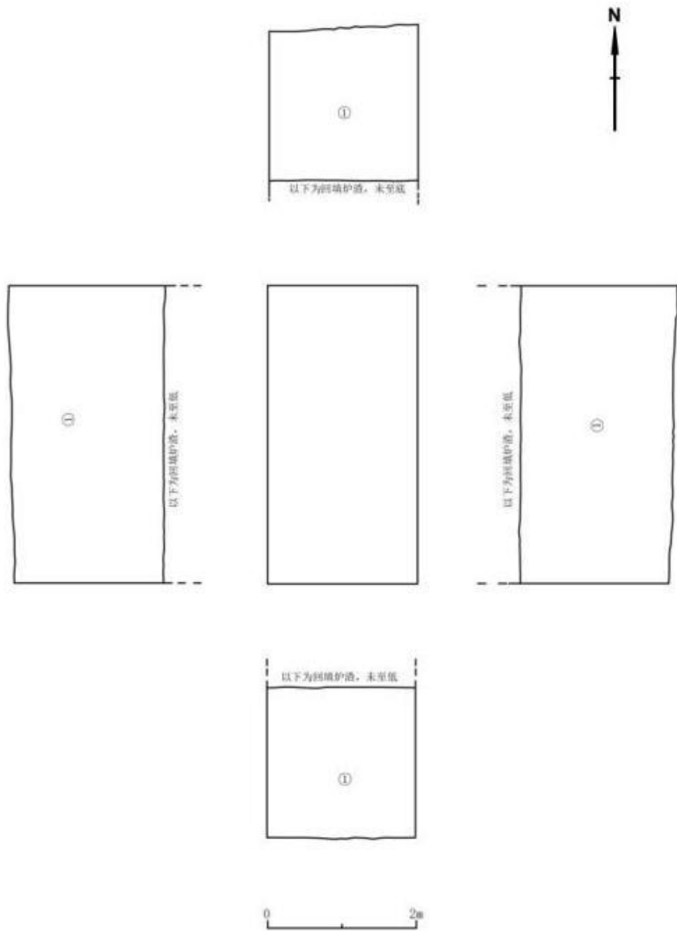
图 77 TG1 平剖面图
