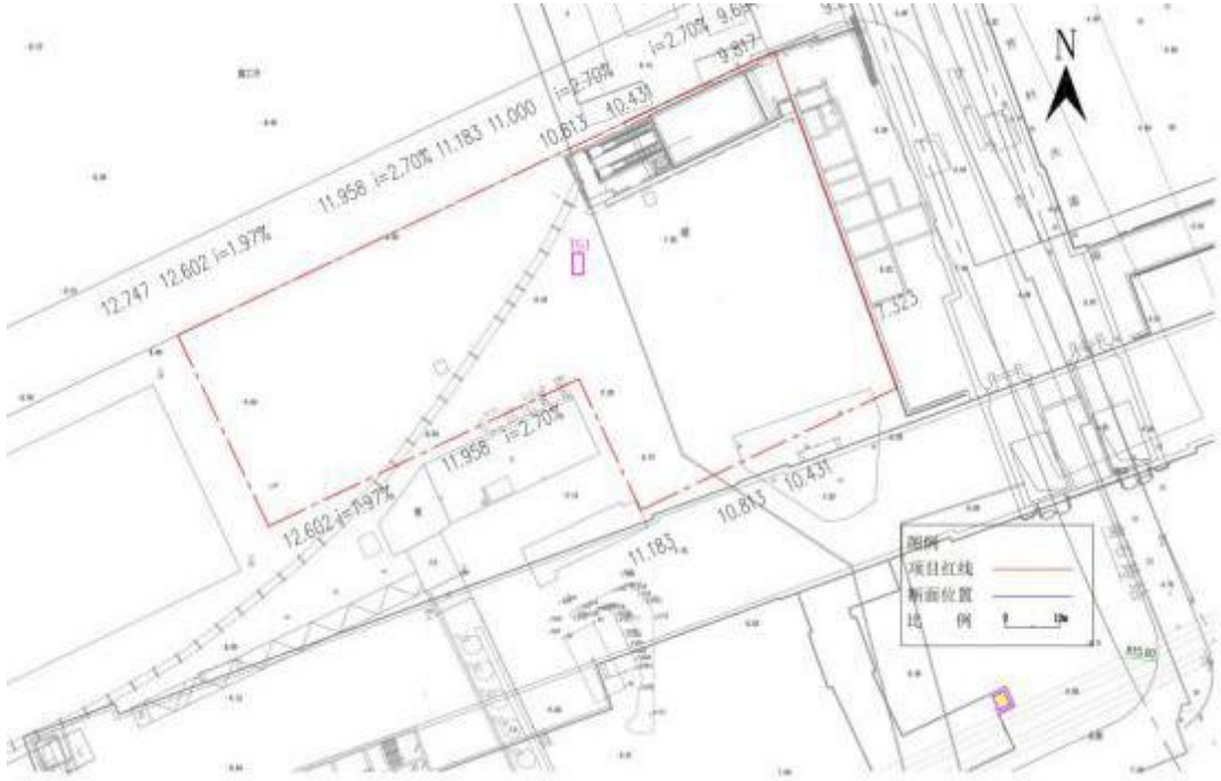
图 60 荔湾区鹤洞东公共人防工程探沟分布示意图（洋红色线范围为探沟）
