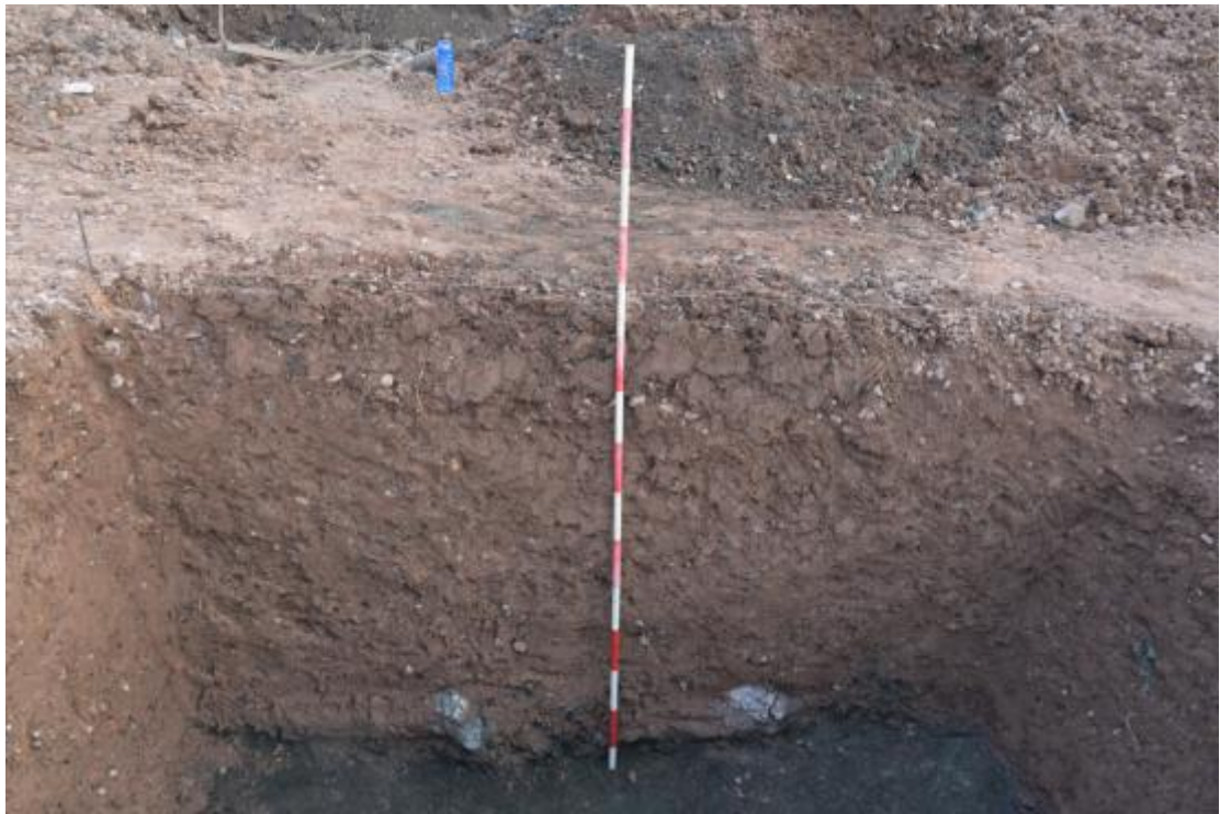
图 73 TG1 东壁剖面（西-东）
