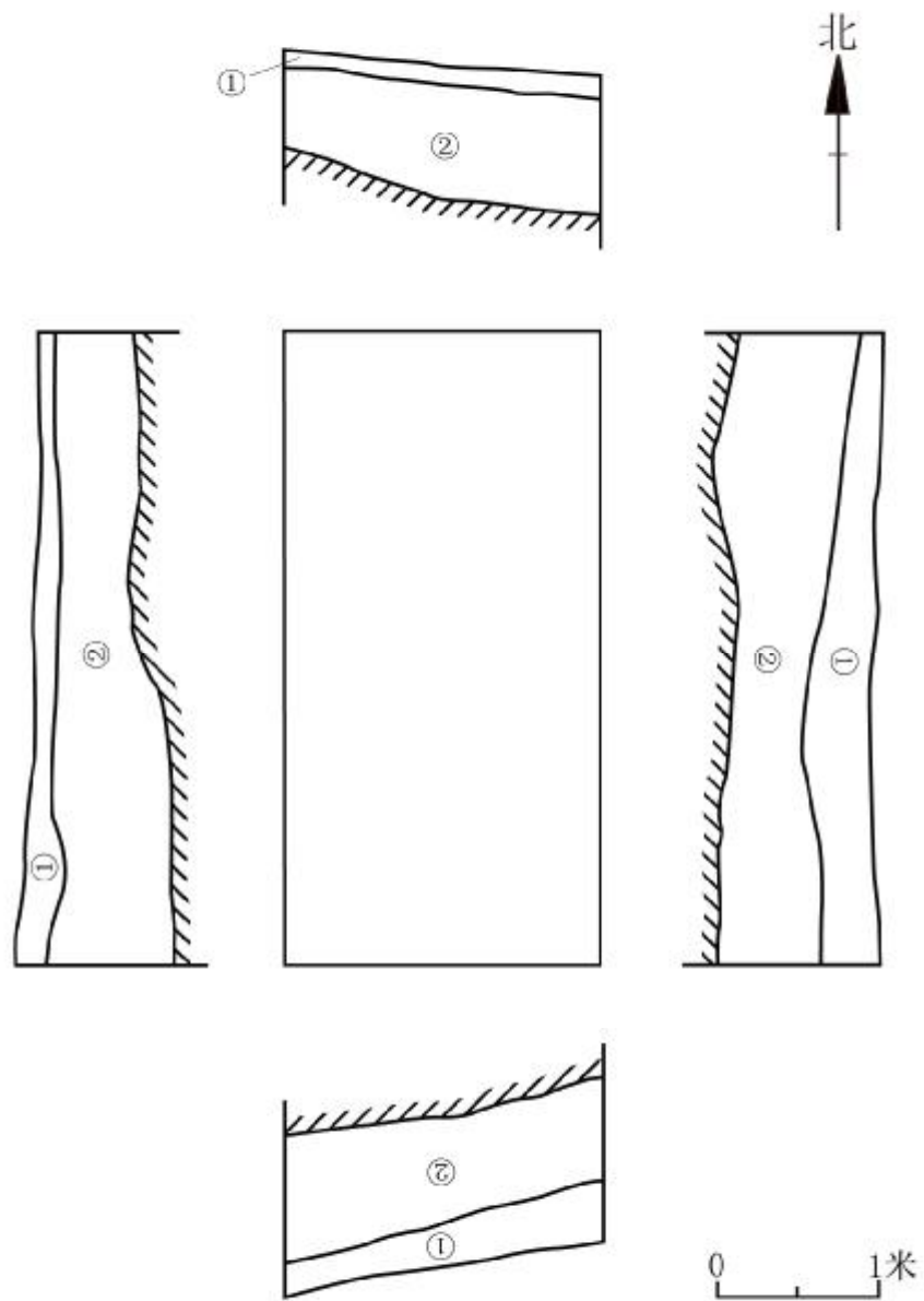
图 66 TG1 平剖面图
